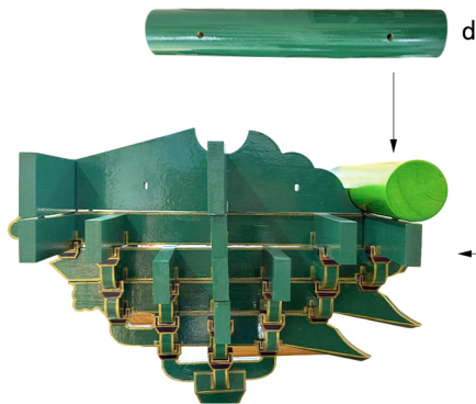
斗拱拼裝完成圖
