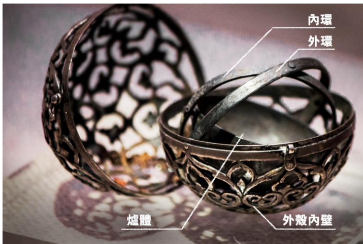
唐代香熏球的構造
