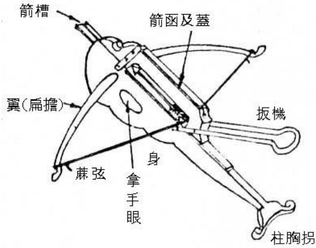
諸葛弩
