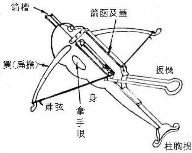
諸葛弩
