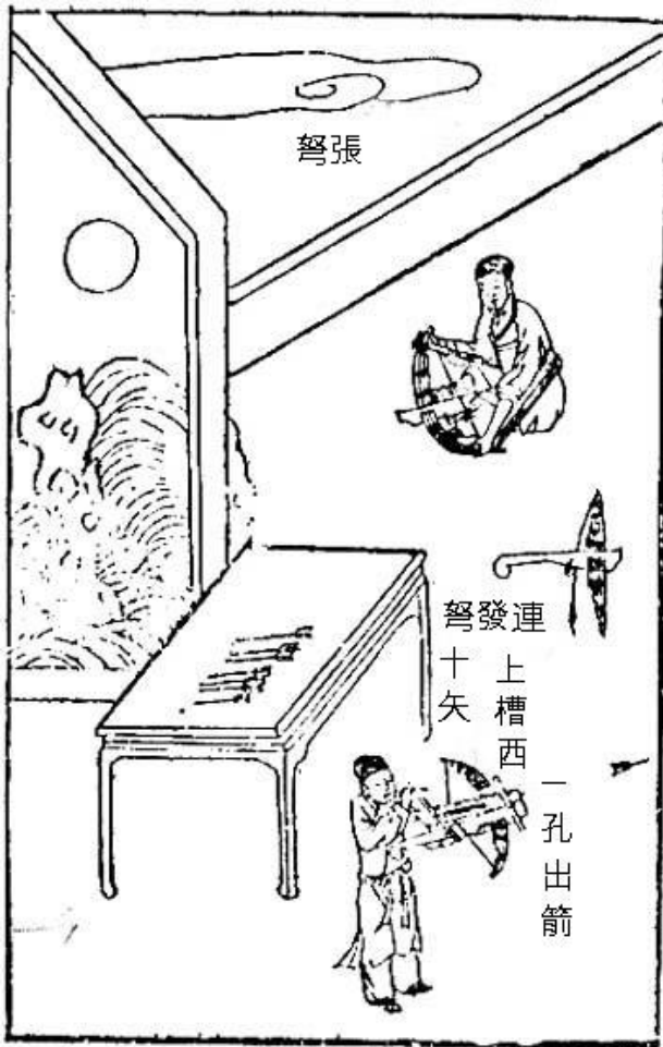
《天工開物》中的連發弩
