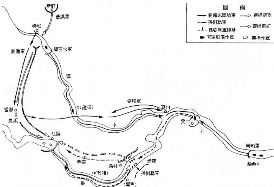
赤壁之戰示意圖
