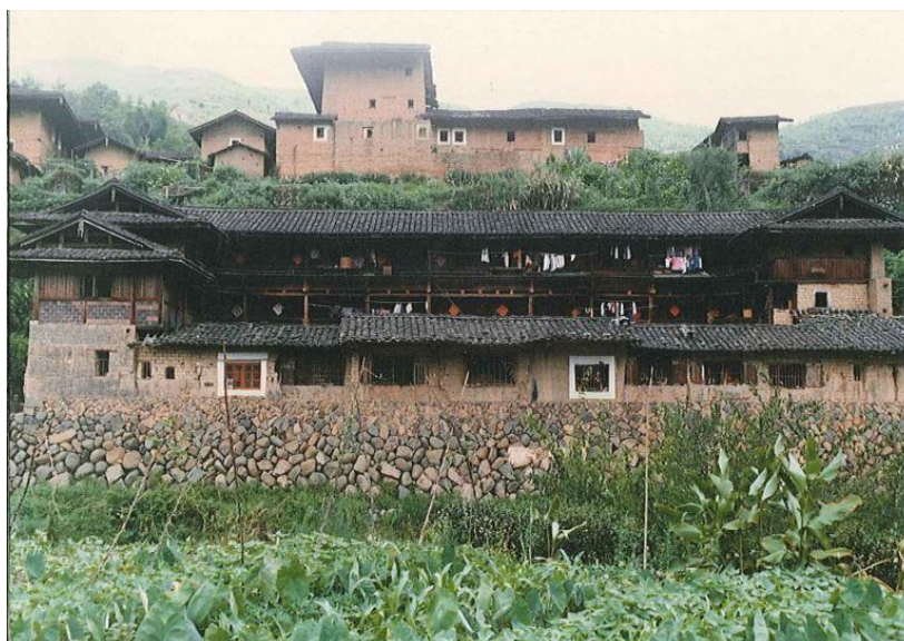
為防水患，土樓多數以大塊卵石築基。
